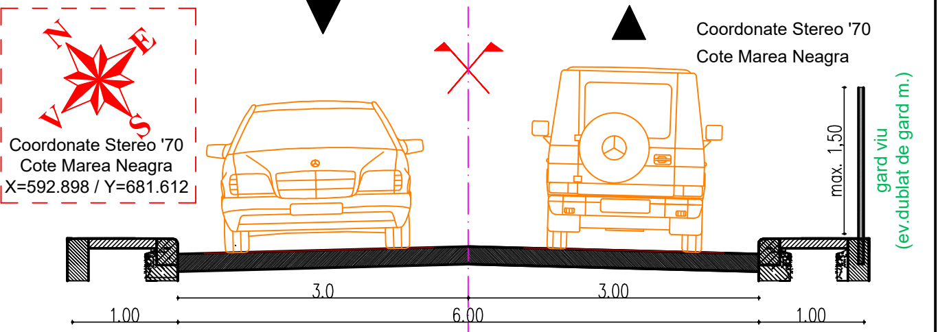
PROFIL TRANSVERSAL ALEE CAROSABILA DE INCINTA
