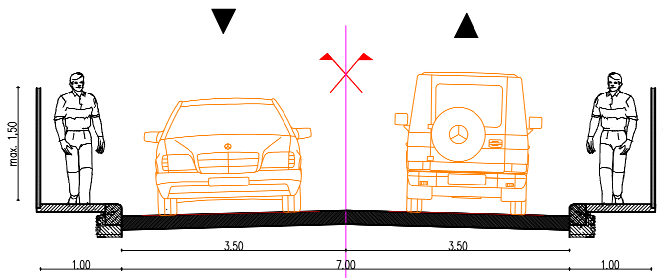
PROFIL TRANSVERSAL DRUM LOCAL POSTERIOR DE ACCES PE PROPRIETATI, EXISTENT, PROPUIS PENTRU MODERNIZARE
