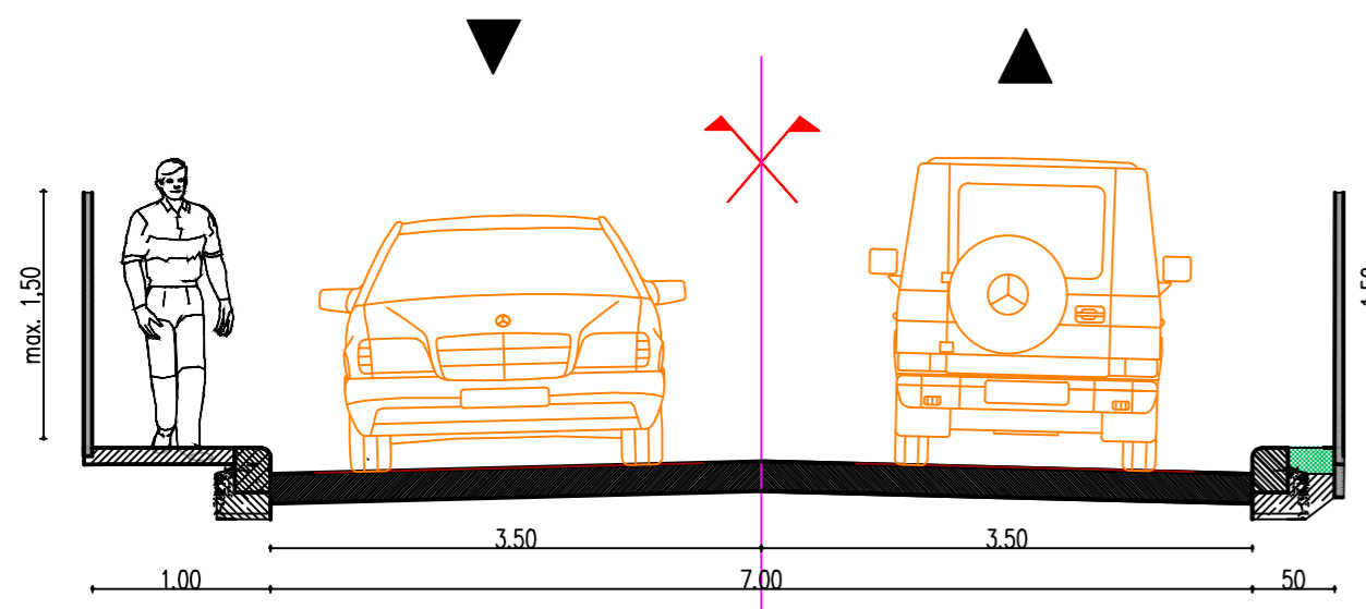
PROFIL TRANSVERSAL STRADA PROPUISA DIN CARE SE FACE ACCESUL PE PROPRIETATI
